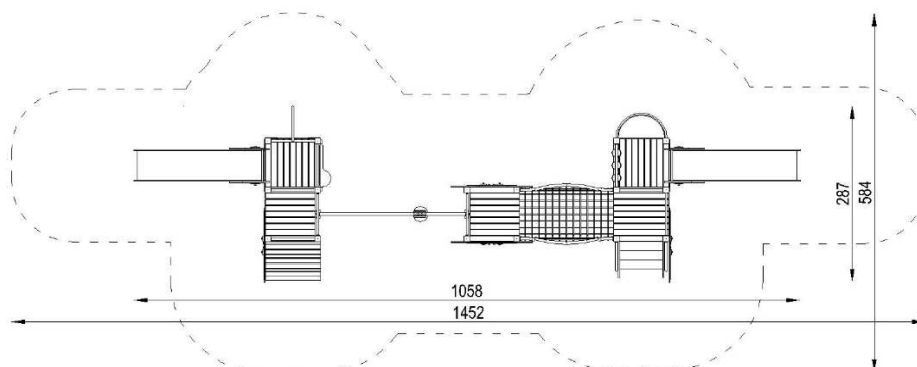
Rzut urządzenia wraz ze strefą funkcjonalną
